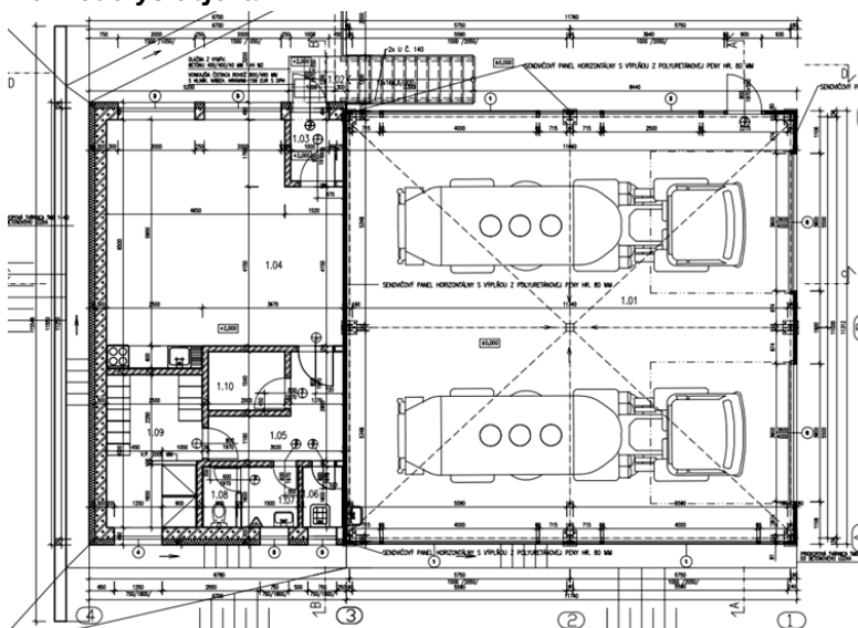
3. Pôdorys objektu
